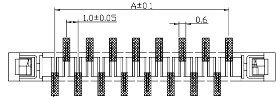
适用线路板 RECOMMENDED PCB LAYOUT
