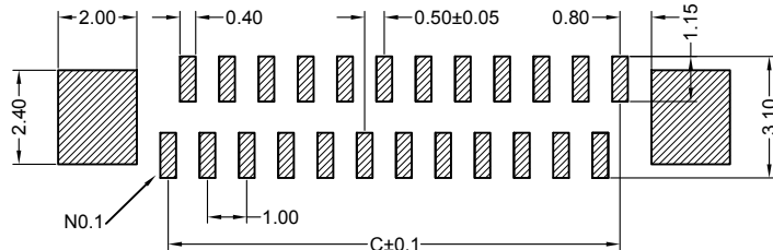
正脚线路板 Positive-needle circuit board
